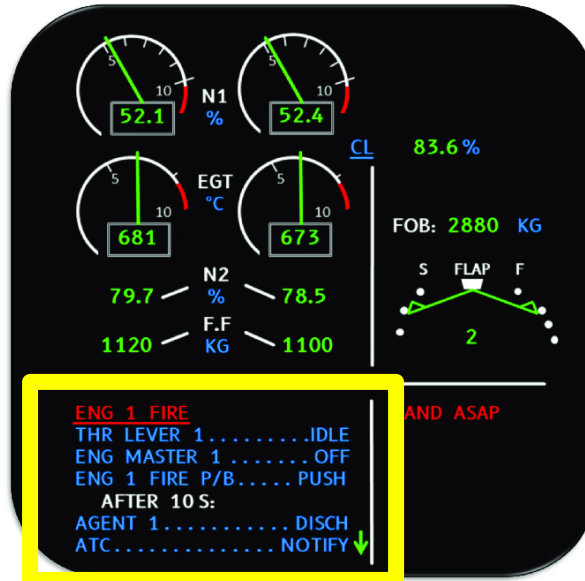
Figura 1 - ECAM do Airbus A320 com procedimentos de fogo no motor
