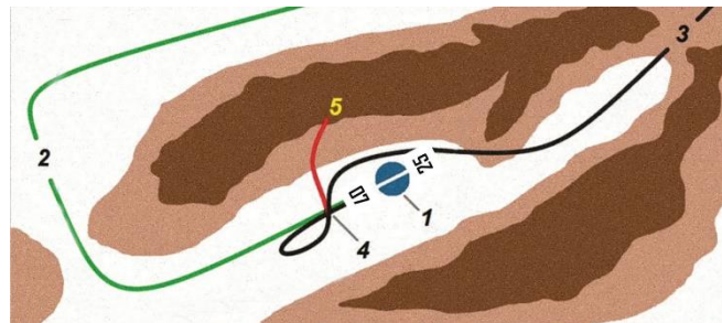
Figura 3 - Procedimentos de saída visual para o aeroporto de Mérida e a trajetória real da aeronave.
